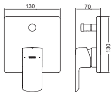
TBN01001B Concealed Box Mini Unit
