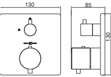
TBN01001B Concealed Box Mini Unit
